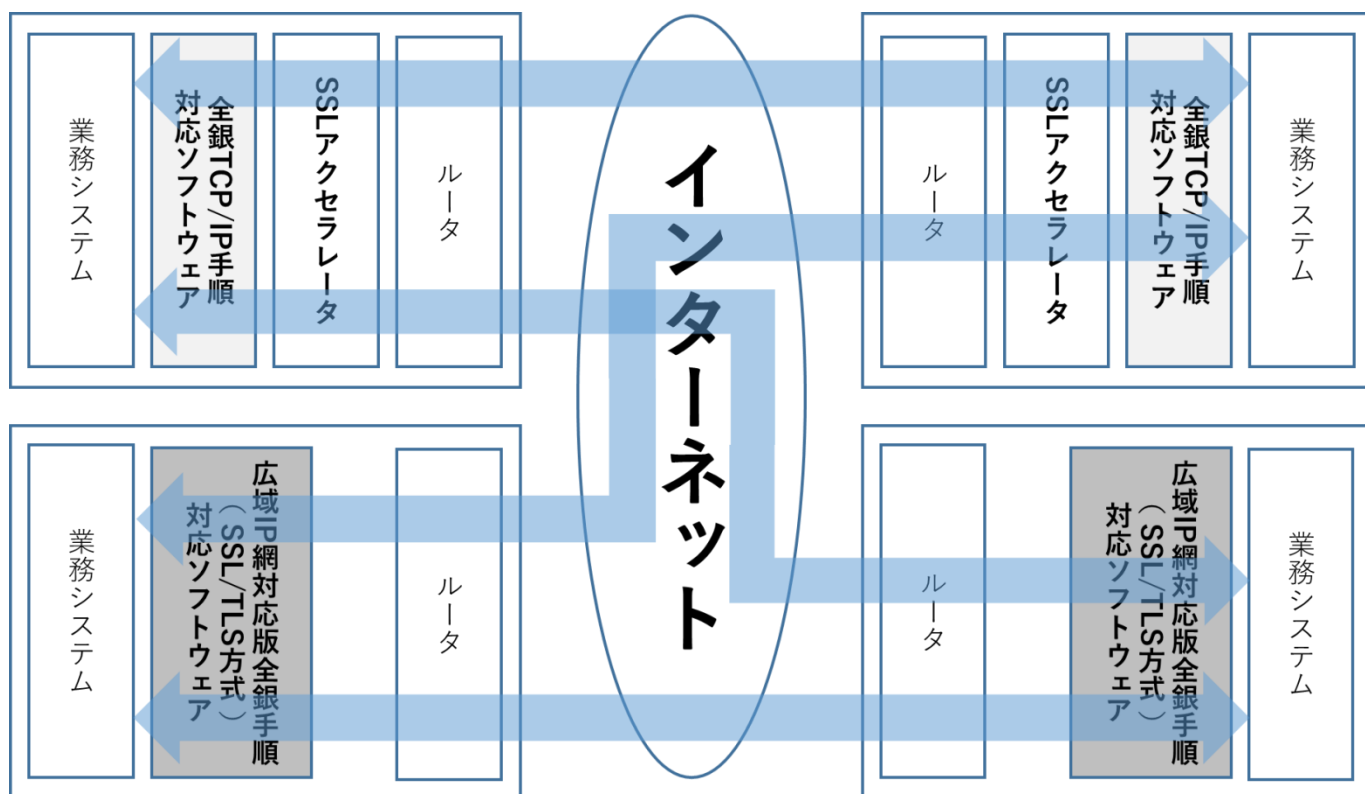
図表 9 SSL/TLS 方式による接続方法
